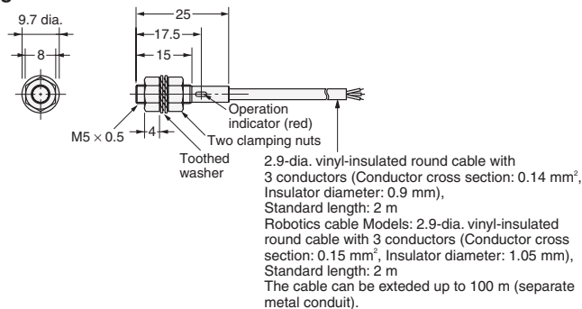
Fig. 3 : E2E-X1□□
