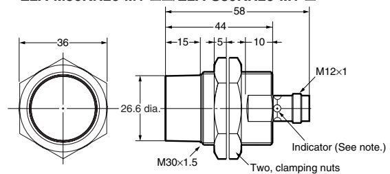
E2A-M30KN20-M1-□□/E2A-S30KN20-M1-□
