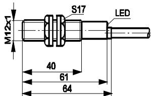
wyjście kablowe
