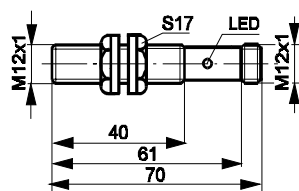
wyjście konektorowe
