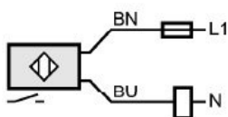
AC NO
